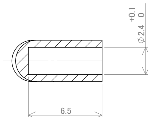
断面図 A-A スケール 5 : 1
